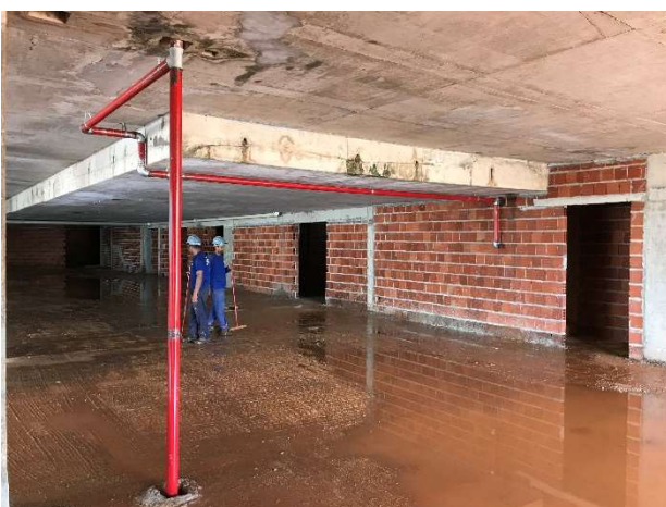
09 – Alvenarias, tubulação de hidrantes, 1ºSS.
