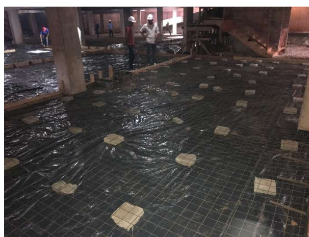
03 – Preparo do piso para concretagem 2º SS.
